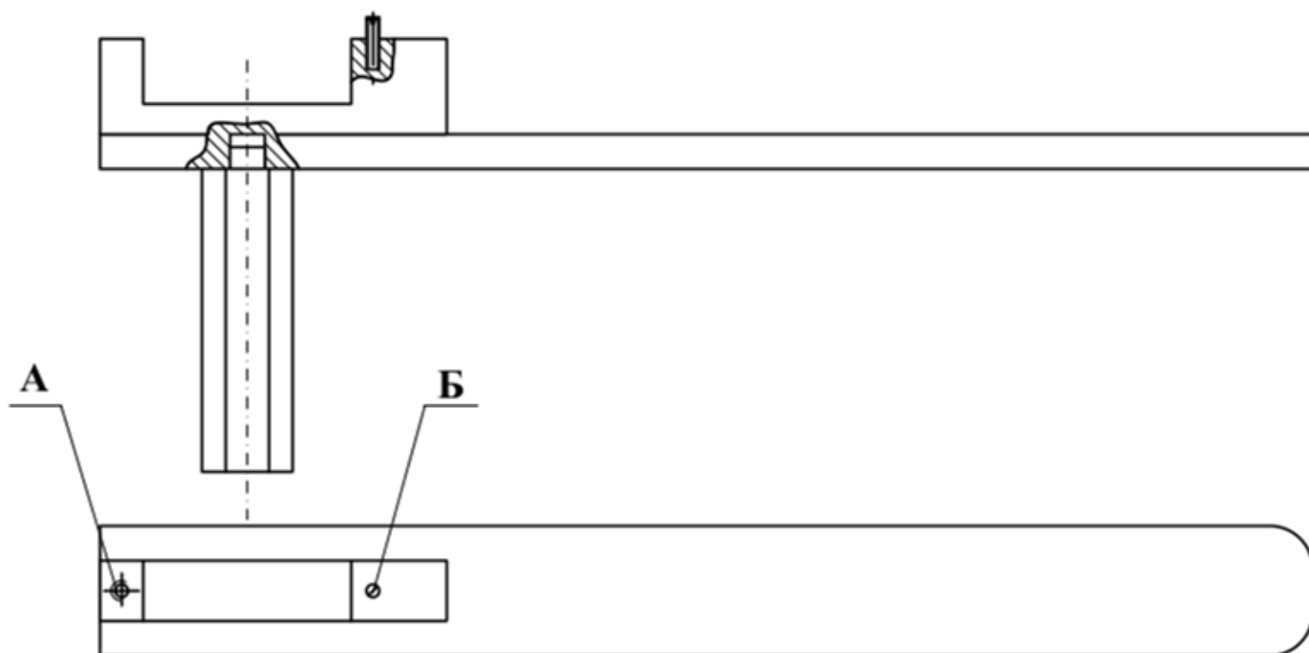
Рисунок А.9 - Ключ КК 2381.04.090
